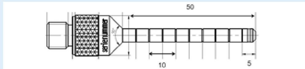
Figuur C2: Specificatie meetpen Specht, maten in mm
