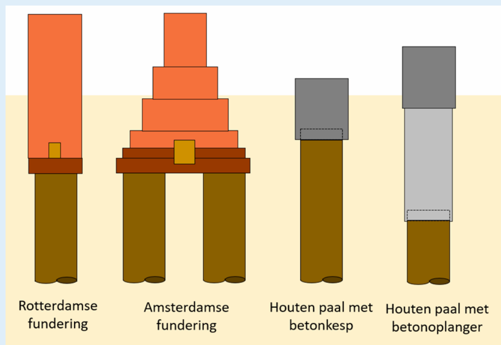
Figuur 7: Funderingstypen in Nederland, A: Rotterdamse fundering, B: Amsterdamse fundering, C: houten paalfundering onder een betonbalk, D: houten paalfundering met betonopzetter (tekeningen KCAF)
